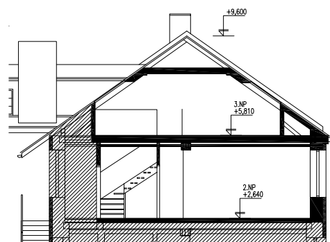
řez M 1:200
